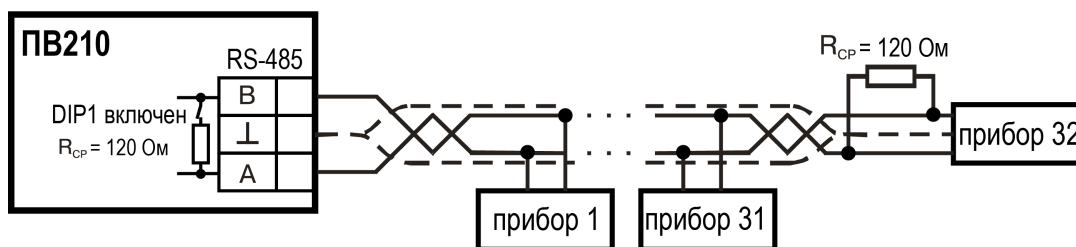
Рисунок 7.2 – Схема подключения
