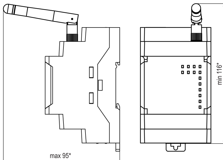
Рисунок 6.2 – Габаритные размеры прибора с подключенной антенной из комплекта поставки
