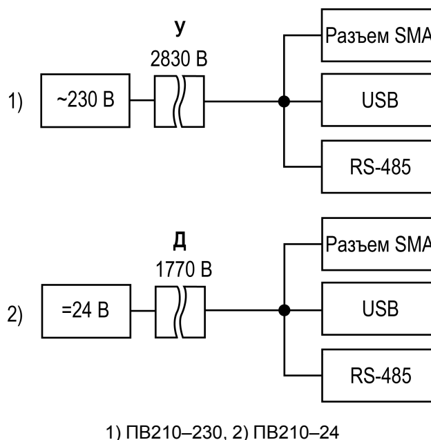
Рисунок 2.1 – Изоляция узлов прибора
