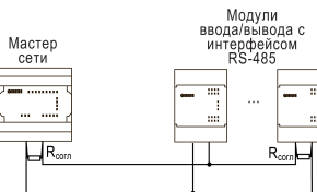
Рисунок 10 – Типовая схема подключения для ПР100 в режиме Master
