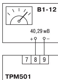
Рисунок 8.5 – Схема подключения
