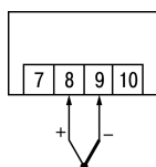
Рисунок 5.4 – Схема подключения ТП
