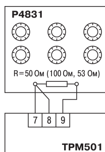
Рисунок 5.3 – Схема подключения
