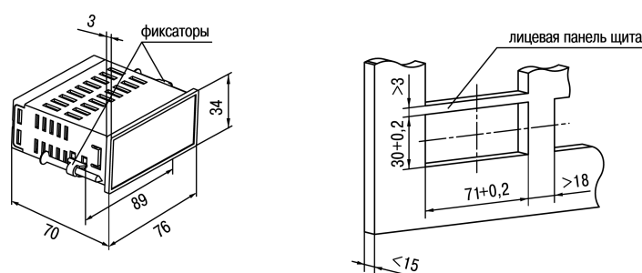
Рисунок 4.2 – Габаритные размеры корпуса ЩЗ
