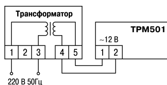
Рисунок 5.6 – Схема подключения трансформатора
