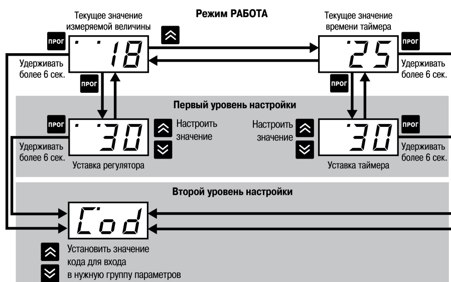
Рисунок 7.1 – Уровни настройки
