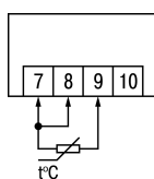
Рисунок 5.2 – Схема подключения ТС
