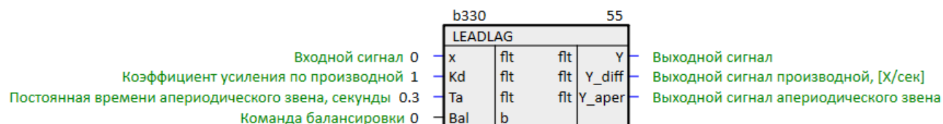
Рисунок 1.37 – Блок компенсации запаздывания сигнала (LEADLAG)
