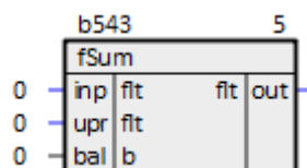
Рисунок 1.6 – Накапливающий сумматор со сбросом и инициализацией (fSum)
