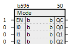
Рисунок 1.22 – Выбор режима (Mode)
