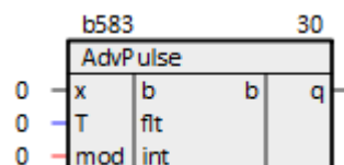
Рисунок 1.18 – Многорежимный генератор импульсов (AdvPulse)
