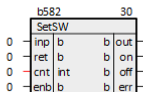
Рисунок 1.17 – Управление реле (SetSW)
