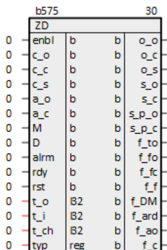
Рисунок 1.13 – Управление задвижкой (ZD)
