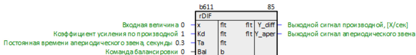
Рисунок 1.31 – Идеальное/реальное дифференцирующее звено с балансировкой (rDIF)
