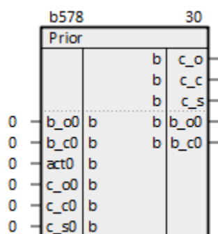
Рисунок 1.14 – Блок приоритетов управления (Prior)
