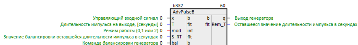
Рисунок 1.32 – Многорежимный генератор импульсов с балансировкой (AdvPulseB)
