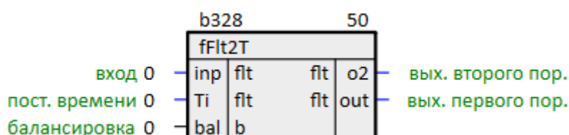
Рисунок 1.36 – Аперидический фильтр 2-го порядка (fFlt2T)
