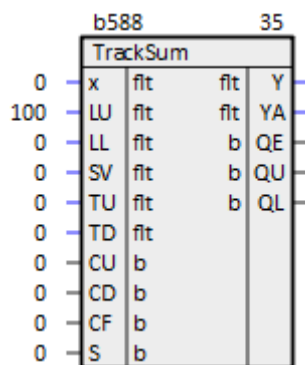
Рисунок 1.19 – Интегрирующий задатчик (TrackSum)
