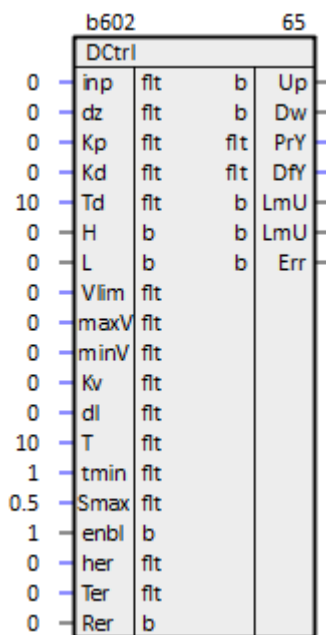
Рисунок 1.25 – Импульсный регулятор (DCtrl)
