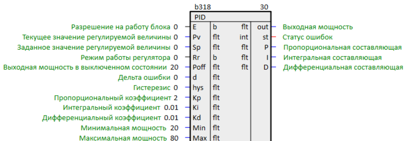
Рисунок 1.27 – ПИД-регулятор (PID)
