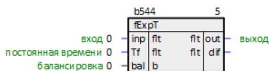
Рисунок 1.8 – Аperiodическое звено (fExpT)
