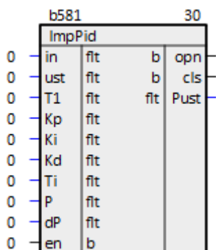
Рисунок 1.16 – Импульсный ПИД (ImpPid)
