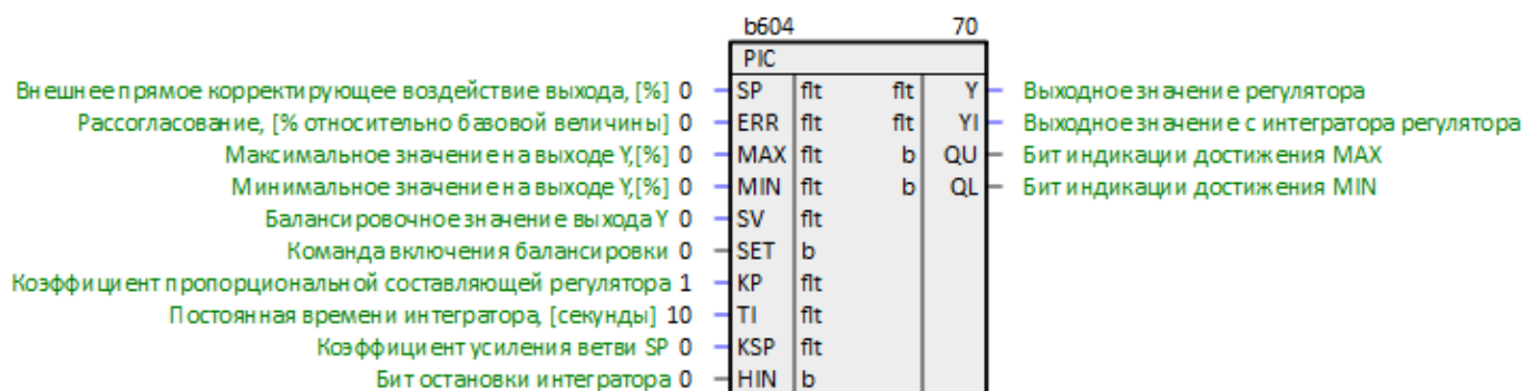
Рисунок 1.26 – ПИ-регулятор (PIC)
