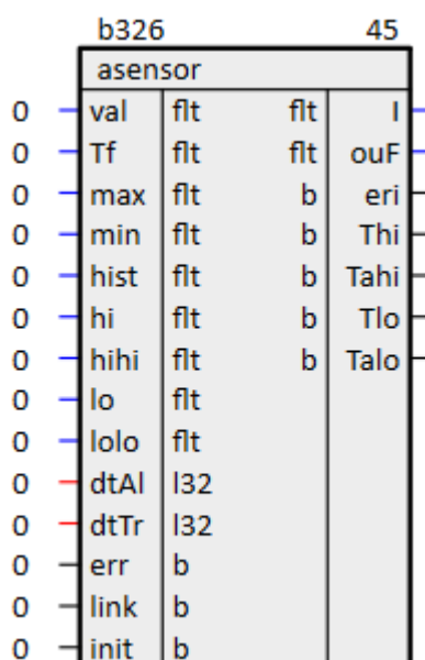
Рисунок 1.35 – Преобразователь 4...20 мА в реальные единицы измерения (asensor)
