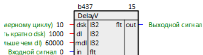
Рисунок 1.5 – Выдача данных с задержкой (DelayV)
