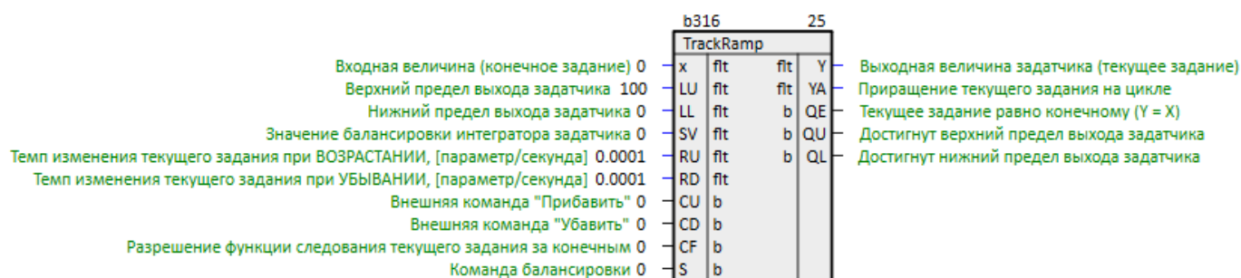
Рисунок 1.30 – Интегрирующий задатчик (TrackRamp)
