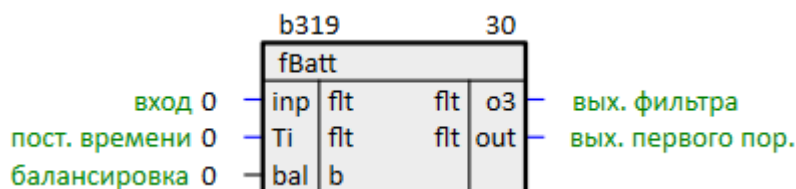
Рисунок 1.33 – Фильтр Баттерворта 3-го порядка (fBatt)
