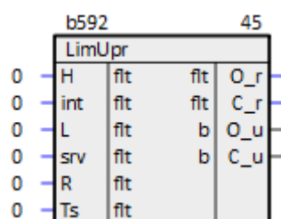
Рисунок 1.21 – Ограничитель ресурсов управления сервоприводом (LimUpr)
