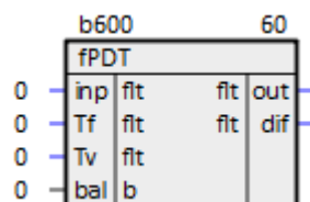
Рисунок 1.24 – ПД-формирователь (fPDT)
