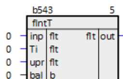
Рисунок 1.7 – Интегратор (flntT)
