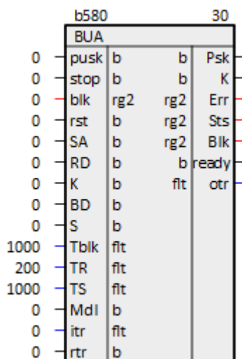
Рисунок 1.15 – Блок управления агрегатом (BUA)
