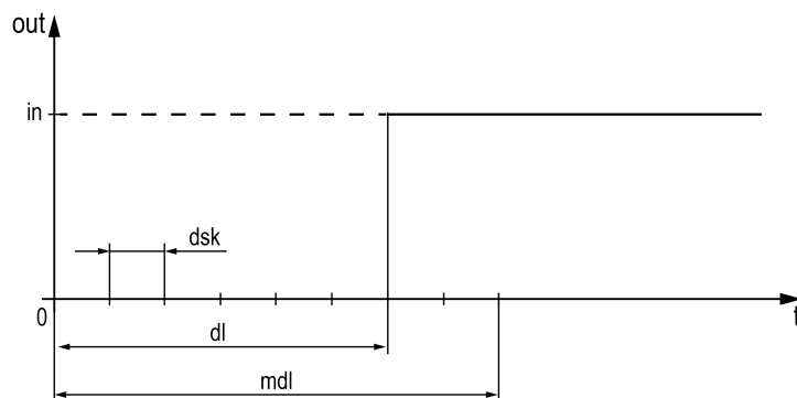
Рисунок 1.4 – Алгоритм DelayV
