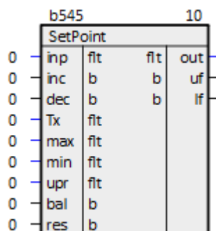
Рисунок 1.9 – Задатчик (SetPoint)
