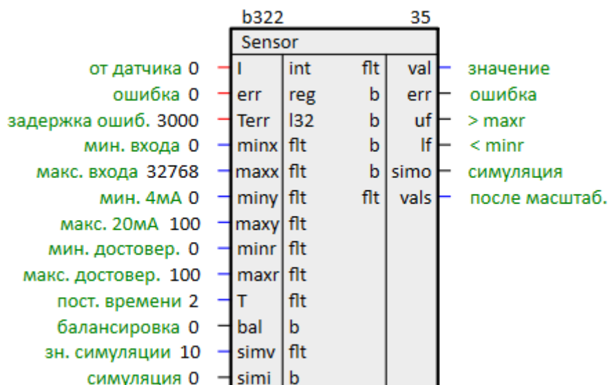
Рисунок 1.34 – Преобразование int-аналоговый вход во float с масштабированием (Sensor)
