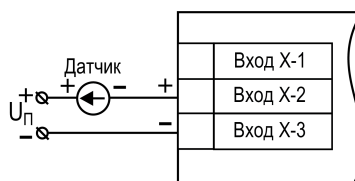
Рисунок 5.20 – Схема подключения пассивного датчика с токовым выходом 0...5 мА или 0 (4)...20 мА
