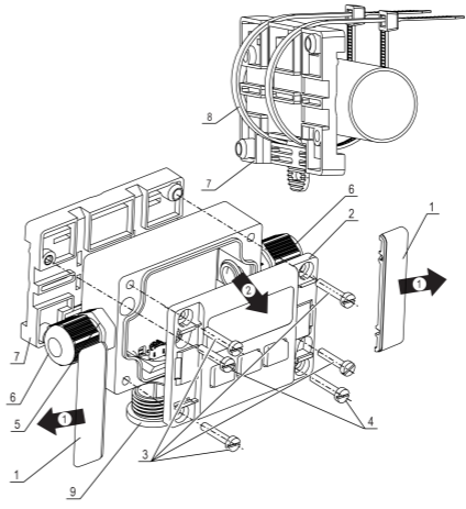
Рисунок 4 – Монтаж прибора
