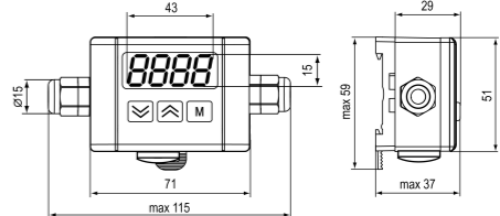
Рисунок 5 – Габаритные размеры корпуса НЗ
