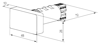
Рисунок 3 – Габаритные размеры прибора
