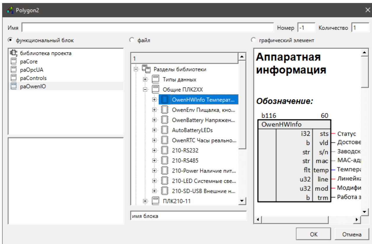
Рисунок 6.6 – Создание блока
