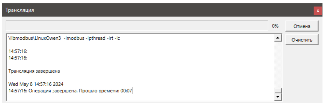
Рисунок 6.11 – Трансляция проекта
