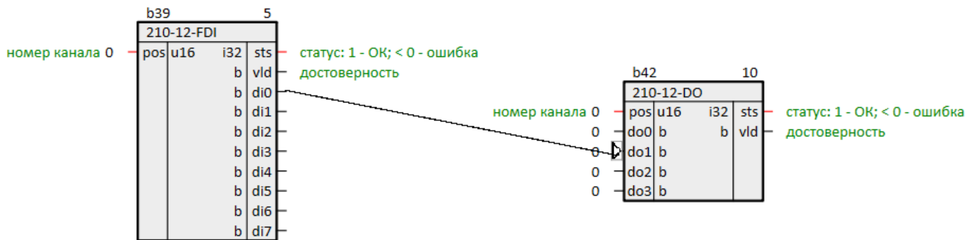
Рисунок 6.9 – Проведение связи
