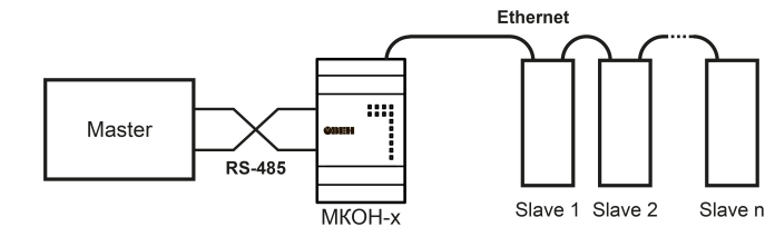
Рисунок 3 – Использование шлюза с Мастером сети в интерфейсе RS-485
