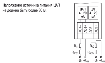
Рисунок 9 – Подключение нагрузки к ВЭ типа «И»
