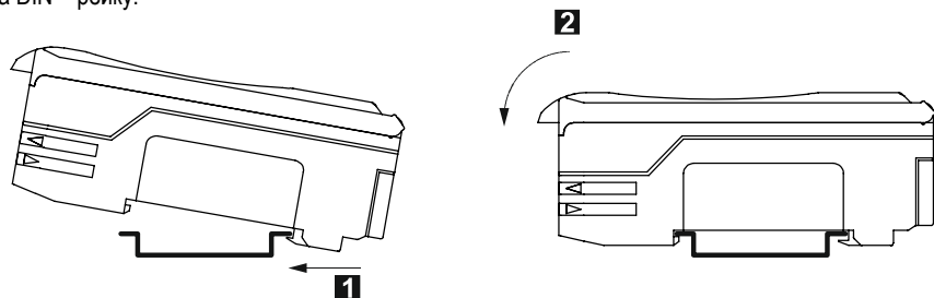
Рисунок 35 – Установка усилителей OF65-UR000FN3.U5.DD/OF65-UR000FP3.U5.DD на DIN-рейку
