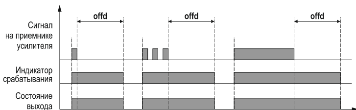
Рисунок 27 – Диаграмма работы усилителя при присвоении параметру ТАИМЕР значения offd
