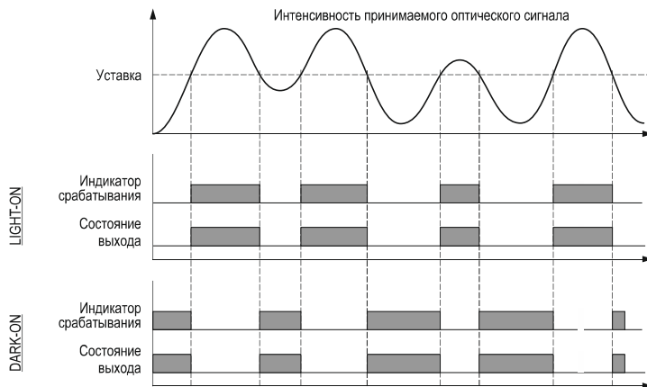
Рисунок 28 – диаграмма состояния выходного ключа усилителя в режиме детектирования Std
