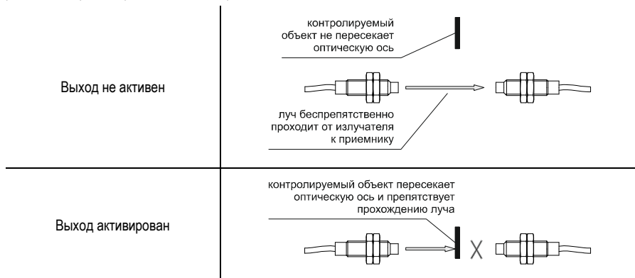
Рисунок 32 – Принцип работы датчика на пересечение луча
