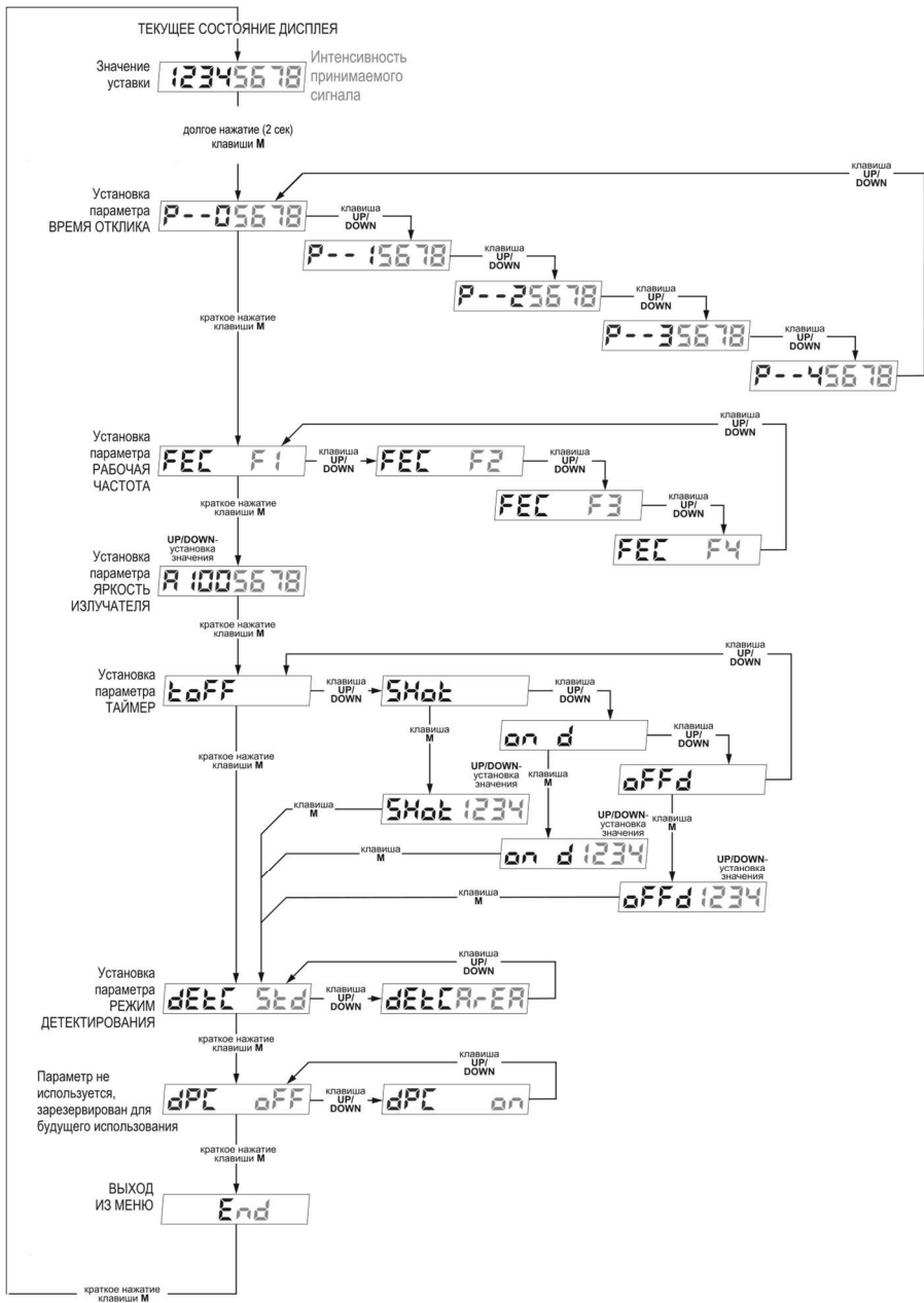
Рисунок 24 – Схема структуры меню усилителей OF65-UR000FN3.U5.K.DD/OF65-UR000FP3.U5.K.DD
