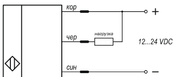
Рисунок 4 – Схема подключения усилителей с NPN – выходом
