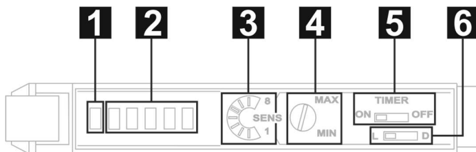
Рисунок 8 – Панель управления усилителей OF65-UR000FN3.U5.K.MD/OF65-UR000FP3.U5.K.MD
