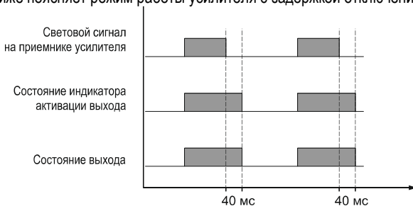
Рисунок 17 – Диаграмма работы таймера в усилителях OF65-UR000FN3.U5.K.MD/OF65-UR000FP3.U5.K.MD
