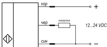
Рисунок 5 – Схема подключения усилителей с PNP – выходом
