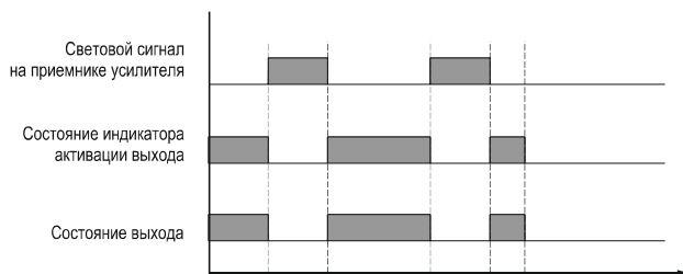
Рисунок 23 – Диаграмма работы усилителей OF65-UR000Fх3.U5.K.DD в режиме на затемнение (DARK-ON)
