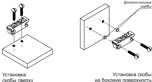
Рисунок 36 – Монтаж установочной скобы
