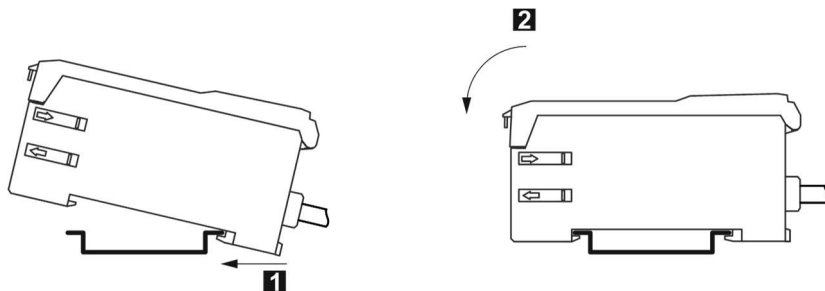
Рисунок 34 – Установка усилителей OF65-UR000FN3.U5.MD/OF65-UR000FP3.U5.MD на DIN-рейку
