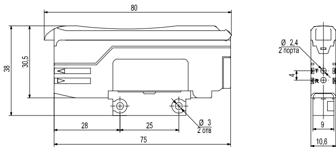
Рисунок 3 - Габаритные и установочные размеры усилителей OF65-UR000FN3.U5.K.DD/OF65-UR000FP3.U5.K.DD
