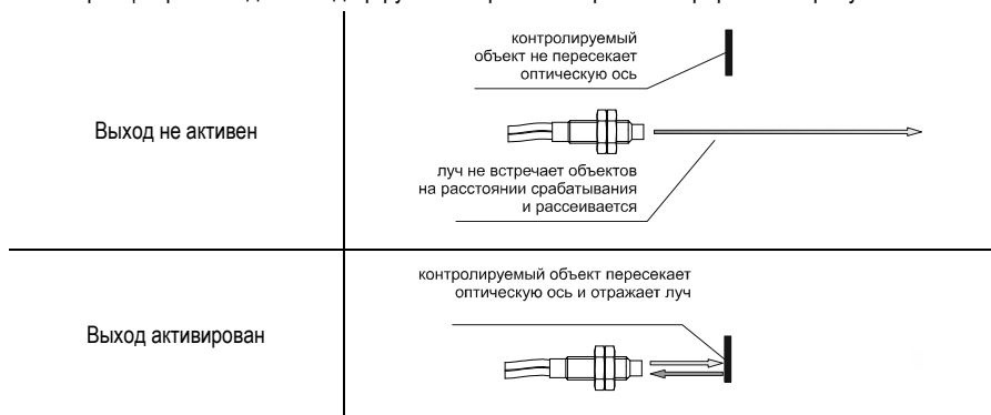
Рисунок 33 – Принцип работы датчика на прием отраженного луча
