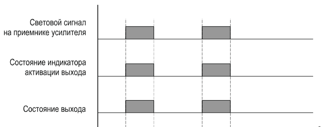
Рисунок 14 – Диаграмма работы усилителей OF65-UR000Fх3.U5.K.MD в режиме на свет (LIGHT-ON)
