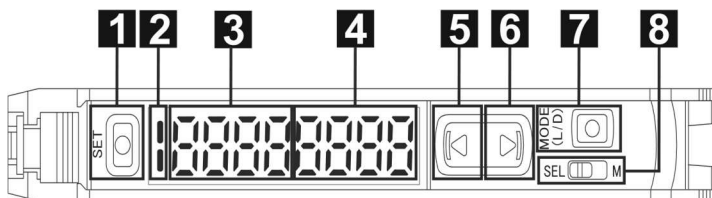
Рисунок 18 – Панель управления усилителей OF65-UR000FN3.U5.K.DD/OF65-UR000FP3.U5.K.DD
