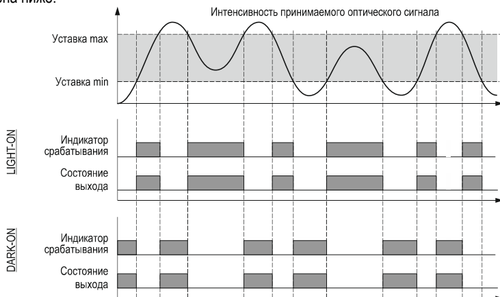
Рисунок 29 - диаграмма состояния выходного ключа усилителя в режиме детектирования ArEA
