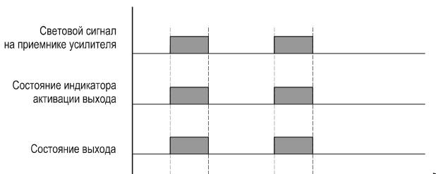
Рисунок 22 – Диаграмма работы усилителей OF65-UR000Fх3.U5.K.DD в режиме на свет (LIGHT-ON)
