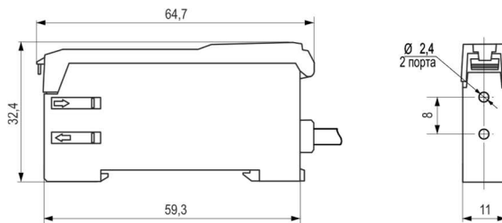
Рисунок 2 – Габаритные и установочные размеры усилителей OF65-UR000FN3.U5.K.MD / OF65-UR000FP3.U5.K.MD
