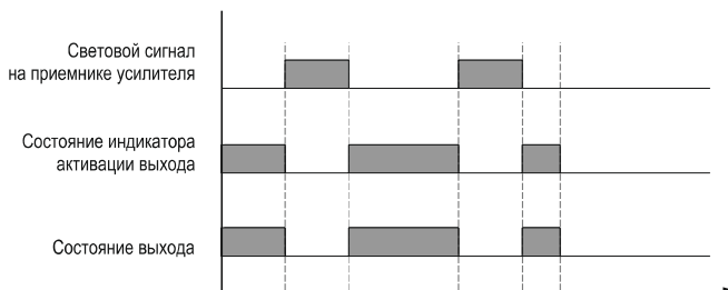
Рисунок 15 – Диаграмма работы усилителей OF65-UR000FN3.U5.K.MD/OF65-UR000FP3.U5.K.MD в режиме на затемнение (DARK-ON)
