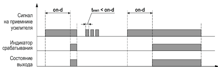
Рисунок 26 – Диаграмма работы усилителя при присвоении параметру ТАИМЕР значения on-d
