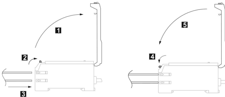
Рисунок 6 – подключение оптоволоконного кабеля и фиксация кабелей в слотах усилителей к усилителям OF65-UR000FN3.U5.K.MD/OF65-UR000FP3.U5.K.MD
