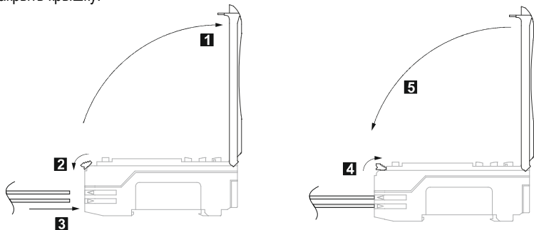
Рисунок 7 - Подключение оптоволоконного кабеля и фиксация кабелей в слотах усилителей к усилителям OF65-UR000FN3.U5.K.DD/OF65-UR000FP3.U5.K.DD
