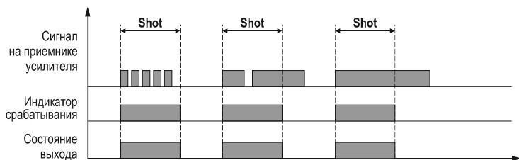
Рисунок 25 – Диаграмма работы усилителя при присвоении параметру ТАИМЕР значения Shot
