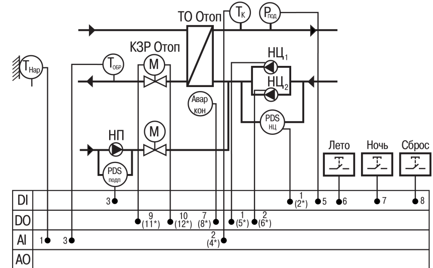
Рисунок 4.1 – Функциональная схема контура «Отопление»
