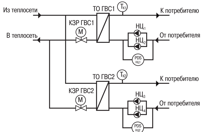
Рисунок 3.5 – Схема контура «ГВС + ГВС»
