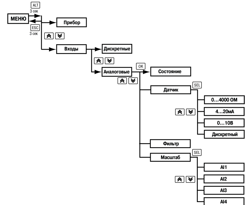
Рисунок 8.5 – Схема системного меню
