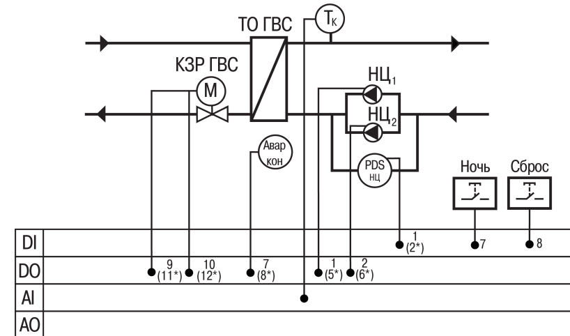
Рисунок 4.2 – Функциональная схема контура «ГВС»
