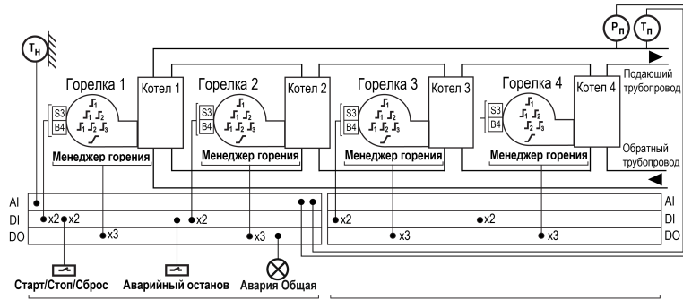
Рисунок 6.1 – Объект управления
